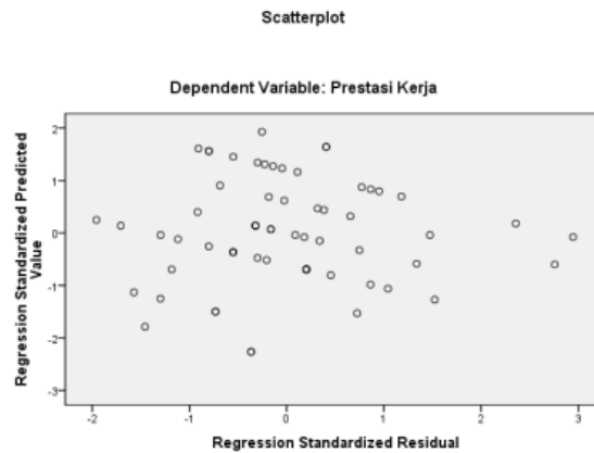
Gambar 1.3 Grafik Scatterplot Hasil Pengujian Heteroskedastisitas
